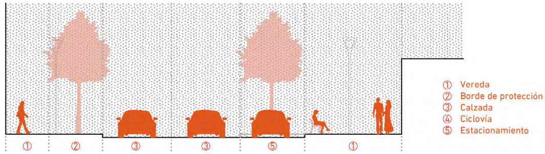
Figura 36_Corte propuesto.
