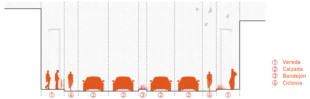
Figura 44_Corte propuesto.
